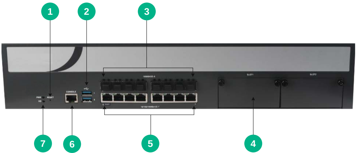
图A-1 UNIS D2000-G20 设备前视图
