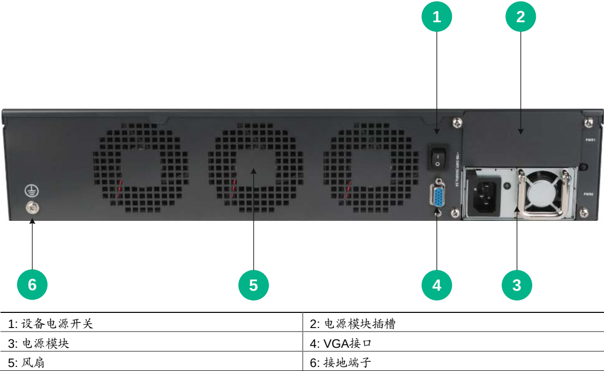
图A-2 UNIS D2000-G20 设备后视图
