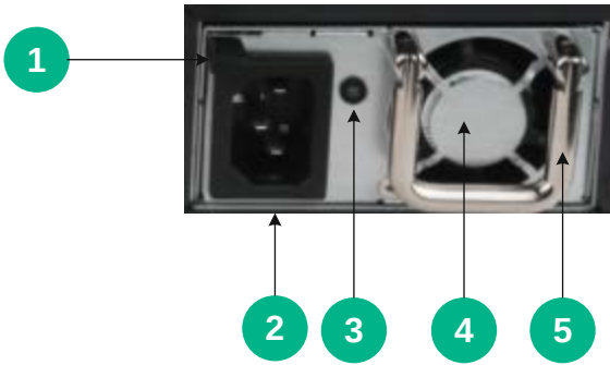
图A-3 R2A-BV0350 交流电源模块正视图
